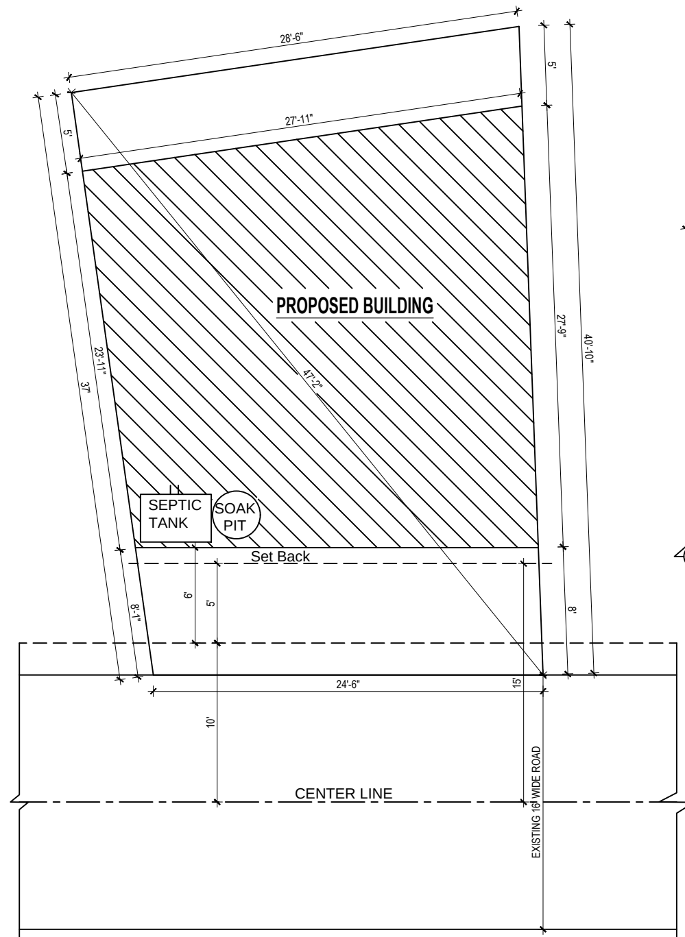
SITE PLAN LAND AREA : 1026.56 SQ.FT. SITE AREA : 1026.56 SQ.FT. PLINTH AREA: 687.75 SQ.FT.
